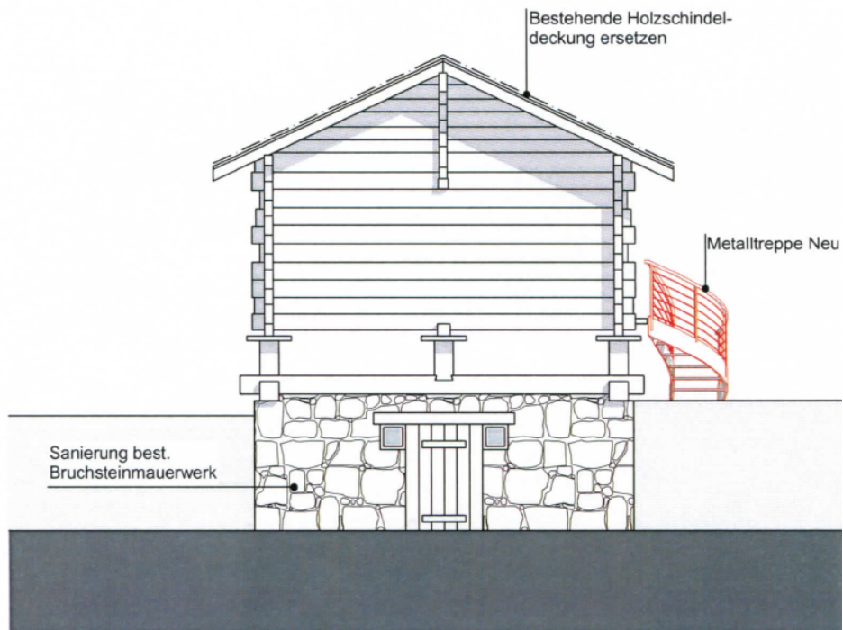
ANSICHT SÜD - WEST
