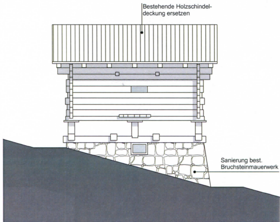
ANSICHT NORD - WEST
