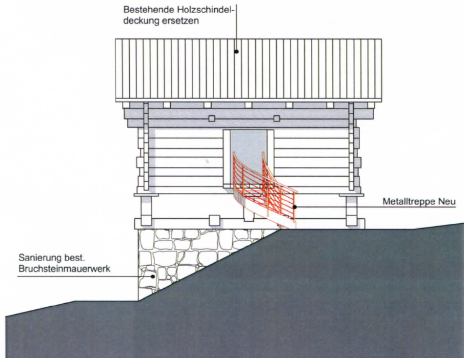
ANSICHT SÜD - OST
